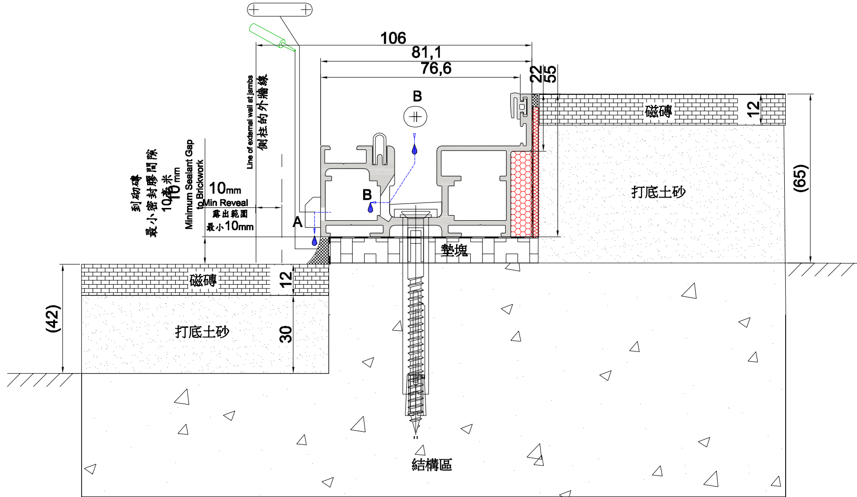
標準門檻施工示意圖 --- 乾式施工
